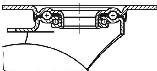
Łożyskowanie wieńca obrotnicy do R1 = 125
