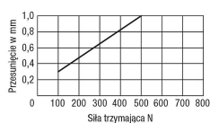
Przesunięcie przy obciążeniu statycznym z jednego kierunku.
